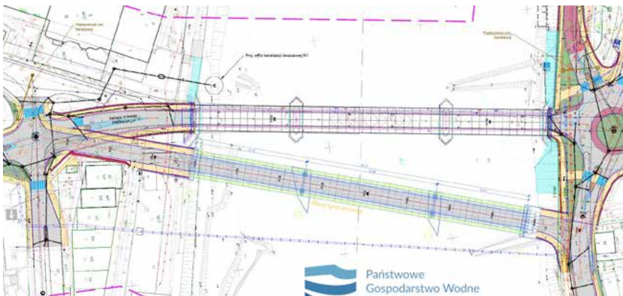
a) Stan projektowany – most tymczasowy
